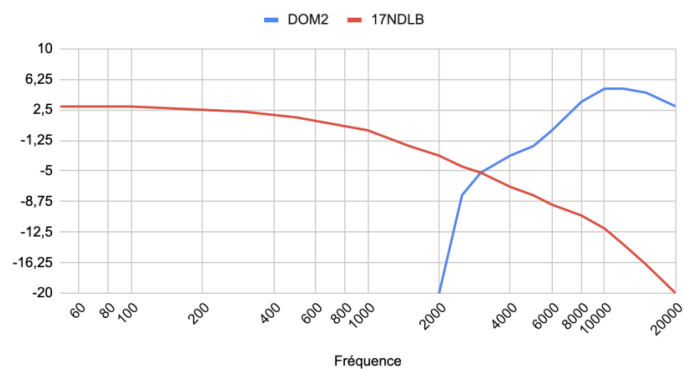
Filtrage Cabasse Galiote M2
