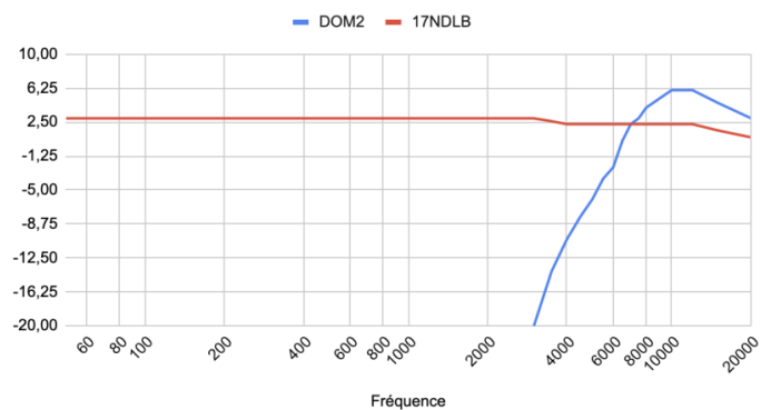
Filtrage Cabasse Galiote M1
